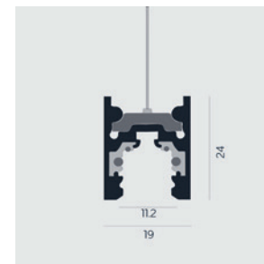
Micro48 Deep - 8650
